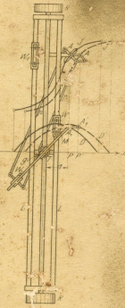
Fig. 27. Der Integrirroll von Alexander Coradi.
